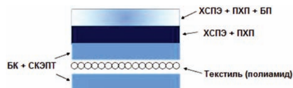
Рис. 2. Структура материала ЛТЛ-1–2.
